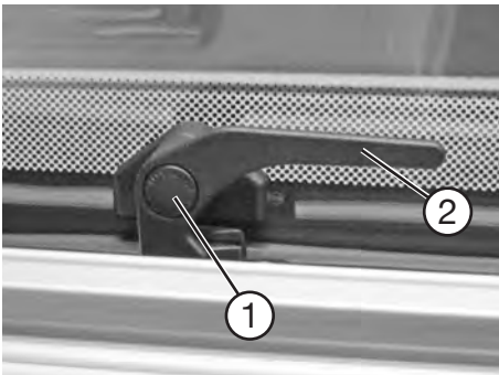
Fensterriegel
