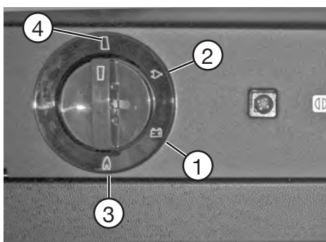
Betriebsarten Kühlschrank
