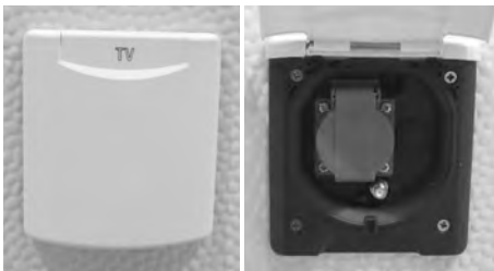
Vorzelt-Außensteckdose mit Antennenanschluss
