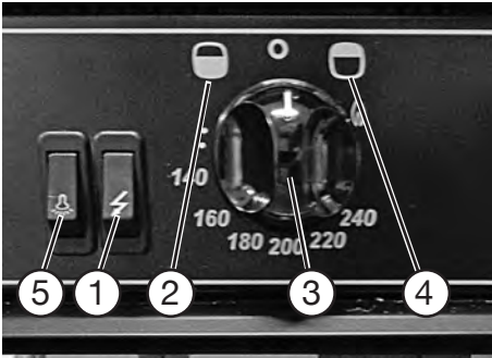
Bedienung Backofen
