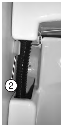
Mechanismus Klappwaschbecken
