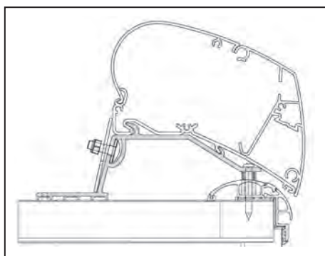
Montage Dachmarkise im Schnitt
